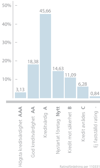
Ratingfördelning i procent på samtliga Sveriges 958 508 aktiva företag
